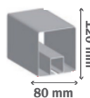
Profil guide 120 x 80
