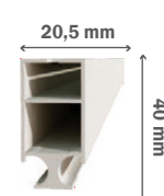
Profil porte toile double
