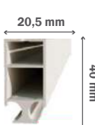
Profil porte toile double
