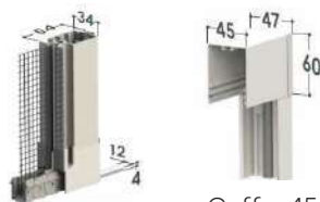
Coffre 45
