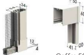
Coffre 50
