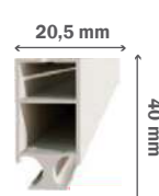
Profil porte toile double
