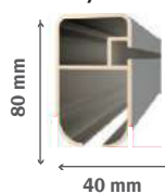
Profil guide
