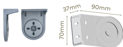
Pose plafond
