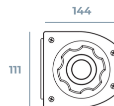
PROFIL COFFRE
